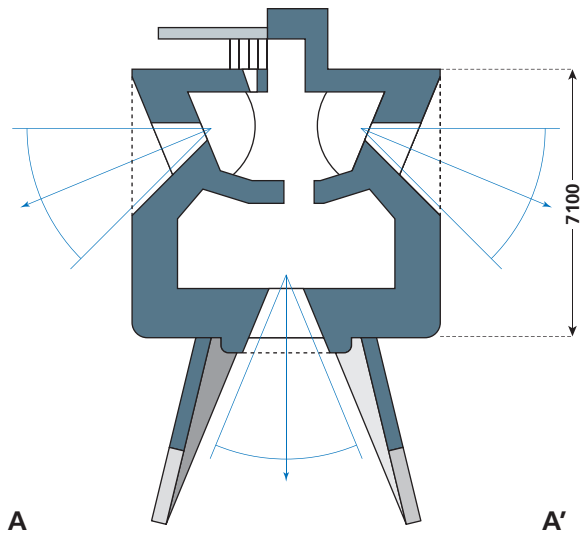
Blockhaus RFM modèle 1935
